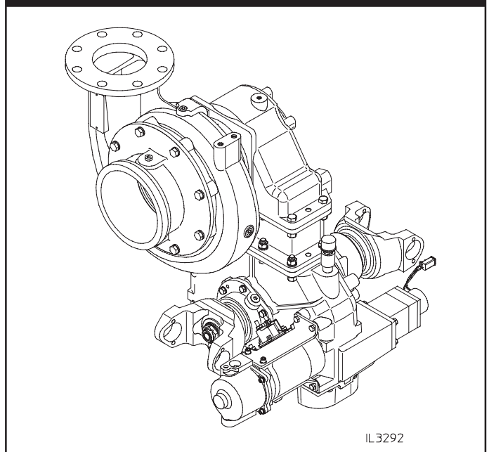
Transmisión C20 montada en la bomba de succión final
