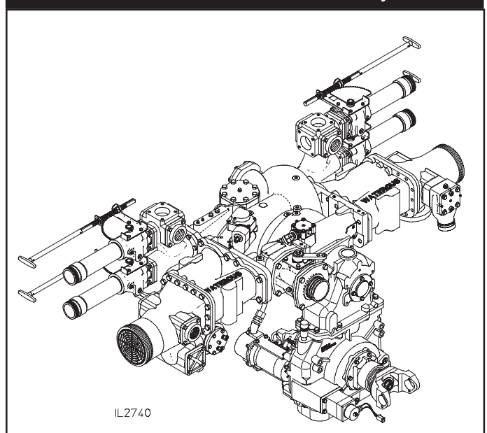
Transmisión C20 montada en bomba de montaje en chasis
