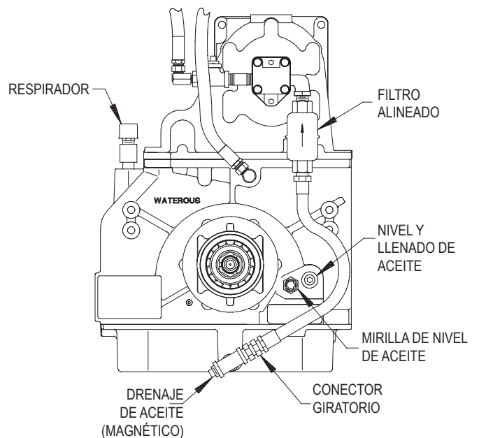
OPCIÓN DE REFRIGERACIÓN EXTERNA DE ACEITE
