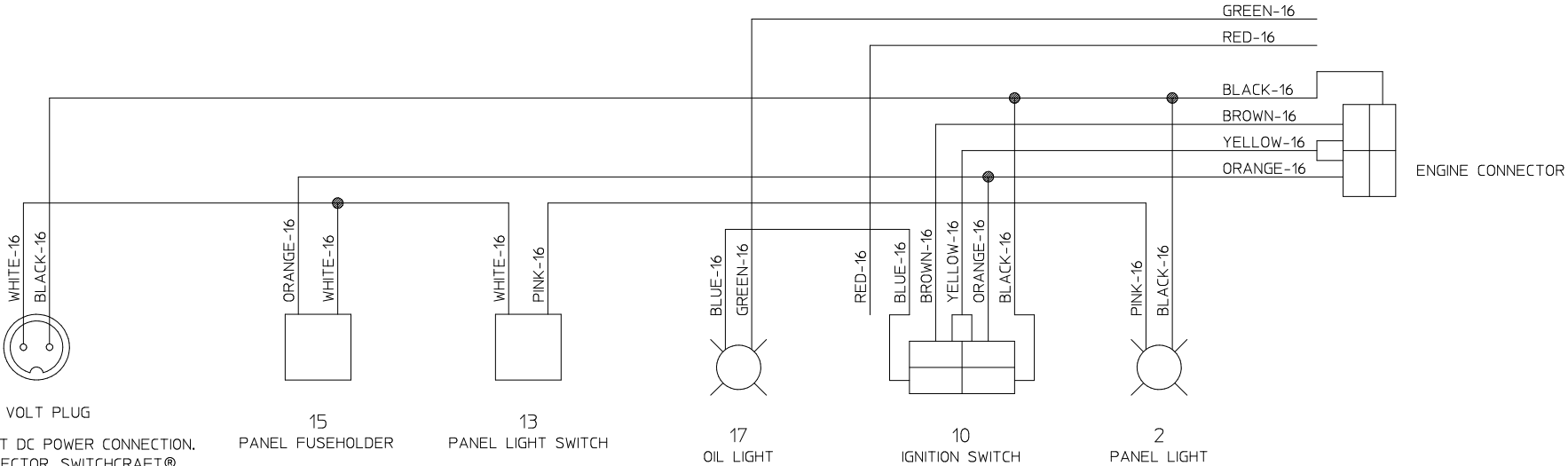
WIRING SCHEMATIC
