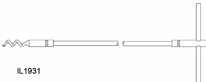
Figura 8. Herramienta de extracción de empaque
