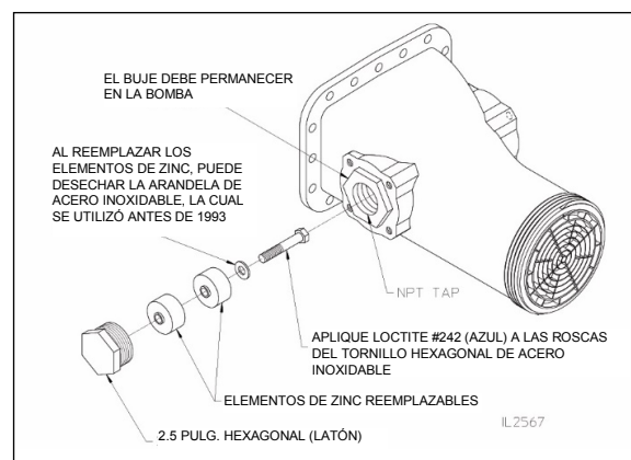
Figura 7. Ánodos roscados
