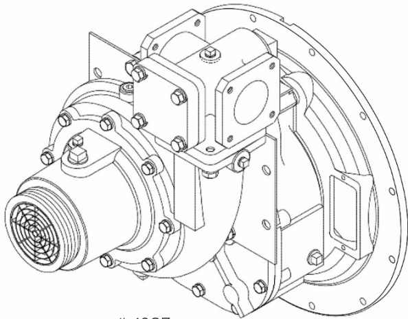
Figura 1. Bomba CLR con transmisión T (montaje directo en motor)
