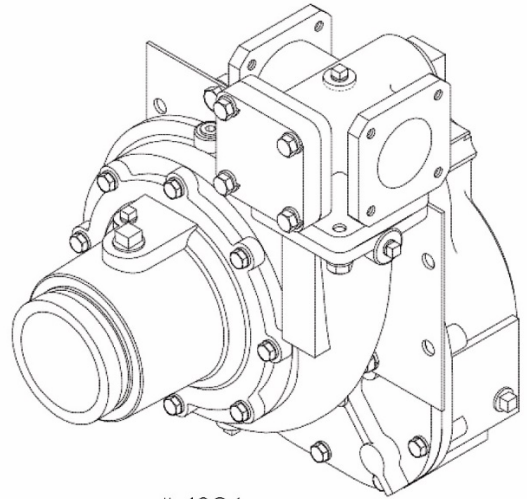
Figura 2. Bomba CLV con transmisión K (impulsada por PTO)
