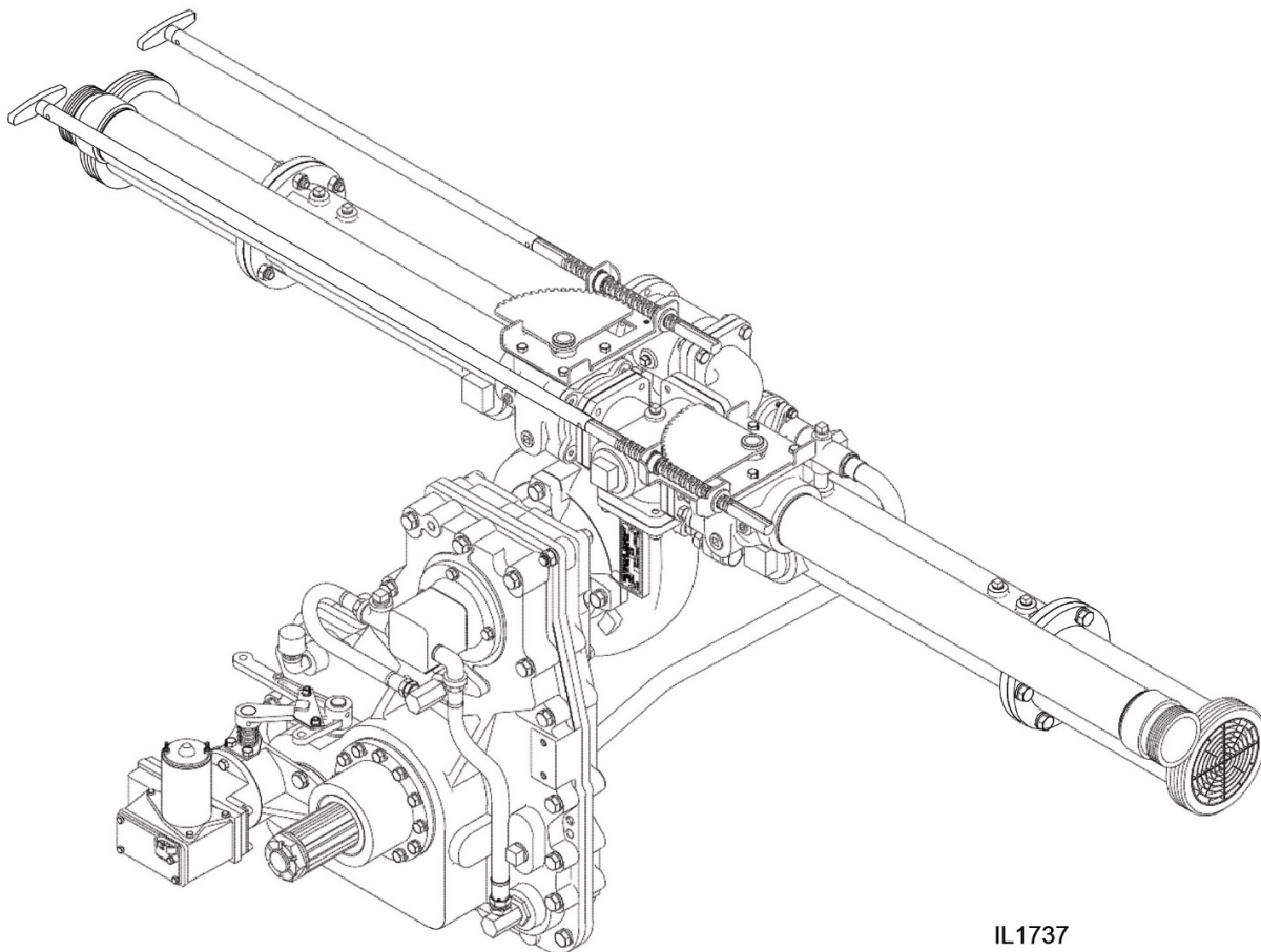
Figura 4. Bomba CLS con transmisión WBX (montaje en el centro) (CLSWBX)
