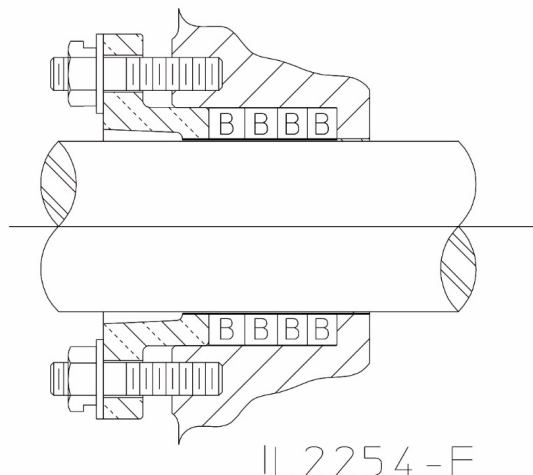
Figura 9. Instalación de empaque y glándula
