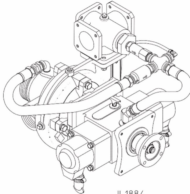
Figura 3. Bomba CLD
